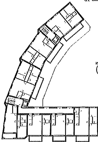
Lokatie Grondplan schaal 1/500
